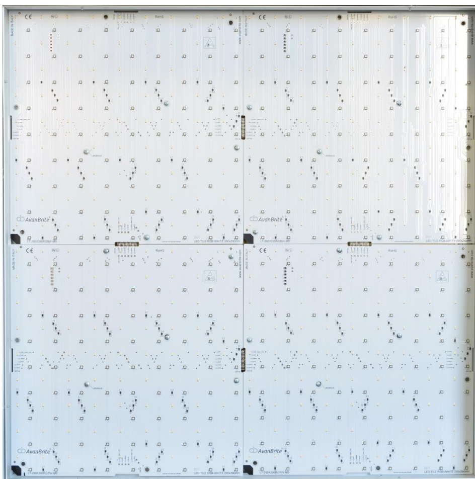
Vista frontale della lampada LED senza lo schermo diffondente
